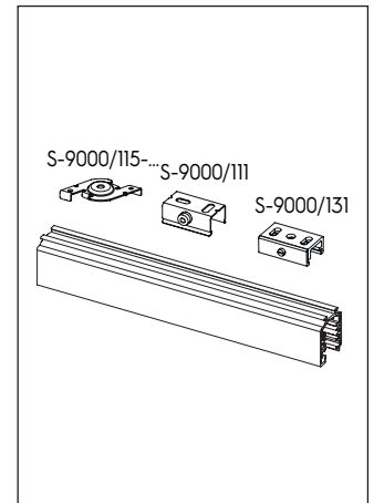
用于轨道两部分间连接的单个配件
