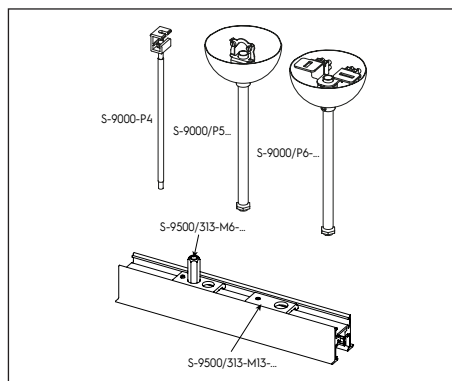
在轨道连接点有调节装置的吊线配件 Suspension sets
