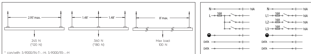
Schema di carico Load scheme
