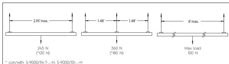
Schema di carico Load scheme
