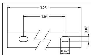
Posizione asole Mounting holes position
